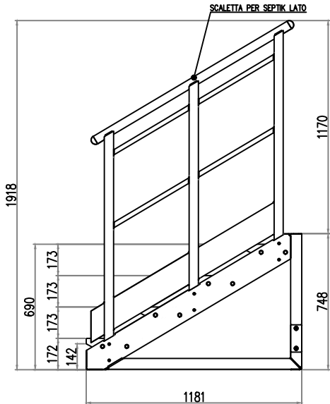
SCALETTA VISTA LATERALE
