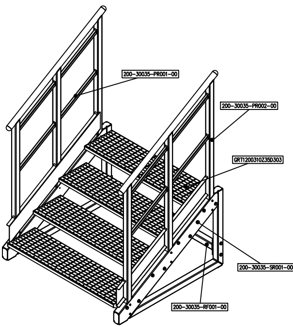
SCALETTA VISTA ASSONOMETRICA
