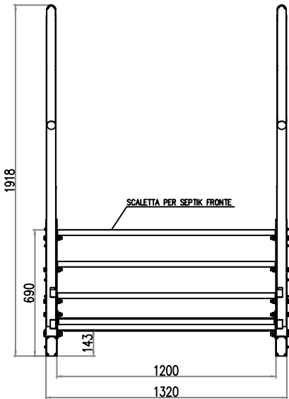
SCALETTA VISTA FRONTALE
